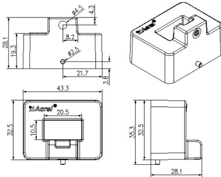
AHKC-BS 霍尔传感器尺寸图
