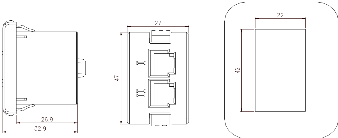
开孔尺寸
