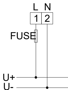
AMB1X0-D(W)-P1 辅助电源
