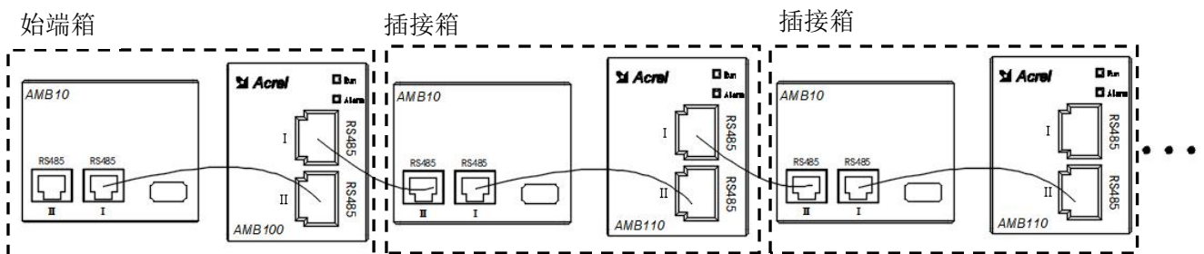
检测模块与显示器连接图
