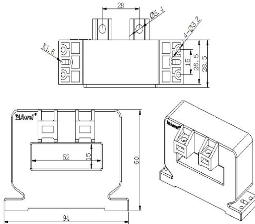
AHKC-FA 霍尔传感器尺寸图
