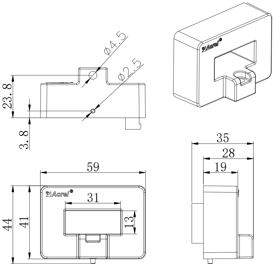
AKH-0.66/W-30NY-250A/100mA 互感器
