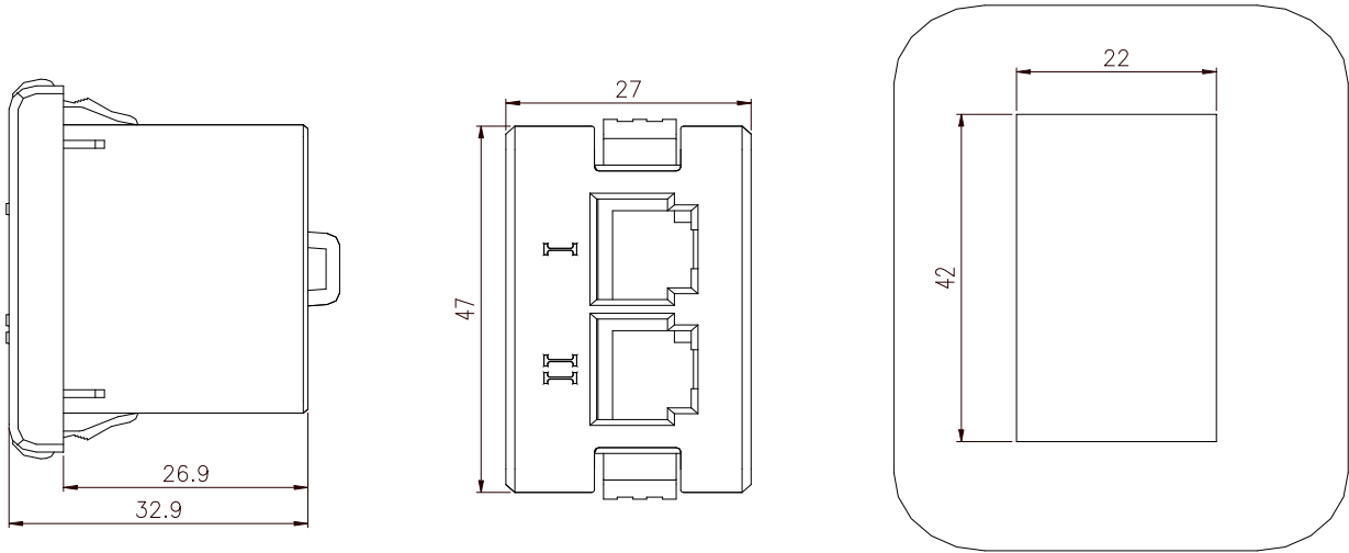
开孔尺寸
