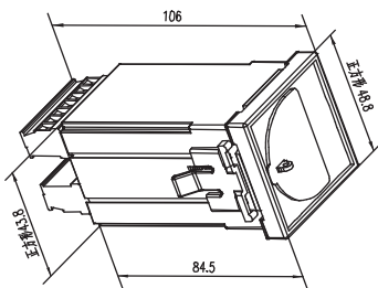
ASJ20 系列外形及开孔尺寸
