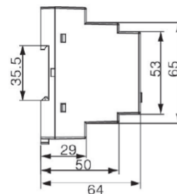
ASJ10 系列外形及安装尺寸
