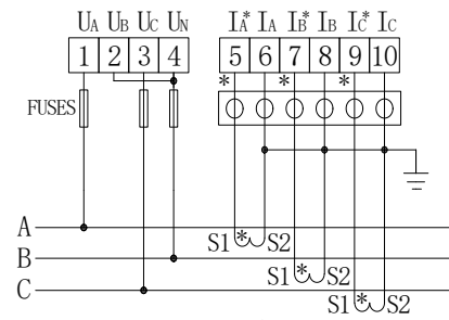
三相三线3CT
