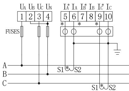
三相三线2CT
